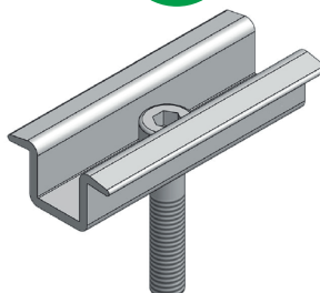
Rahmenmittelklemme - RMK
