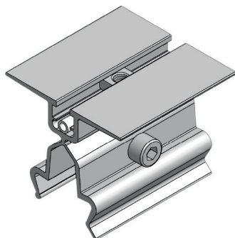
Grundklemme - AGK2
